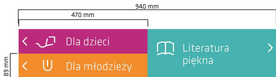
tabliczka nr 1, skala 1:5
